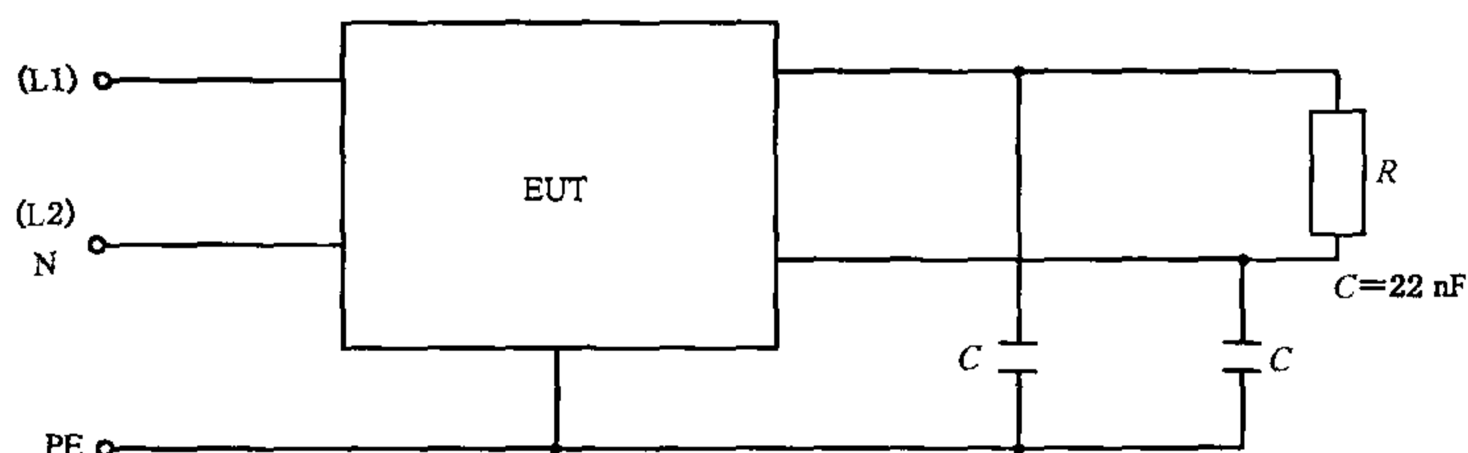
图 L.1 负载故障
