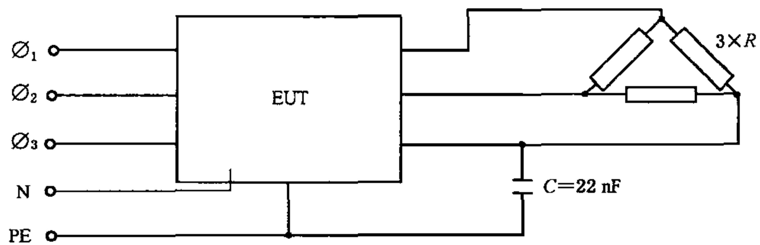
图 L. 1 (续)
